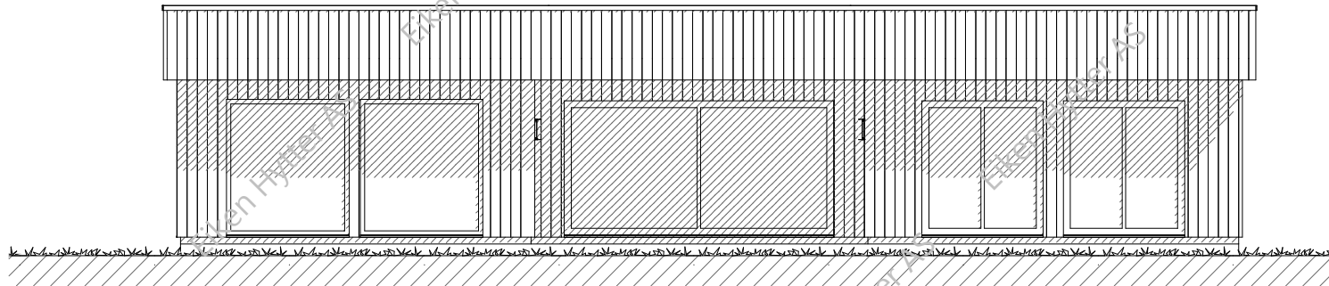
Fasade 1
