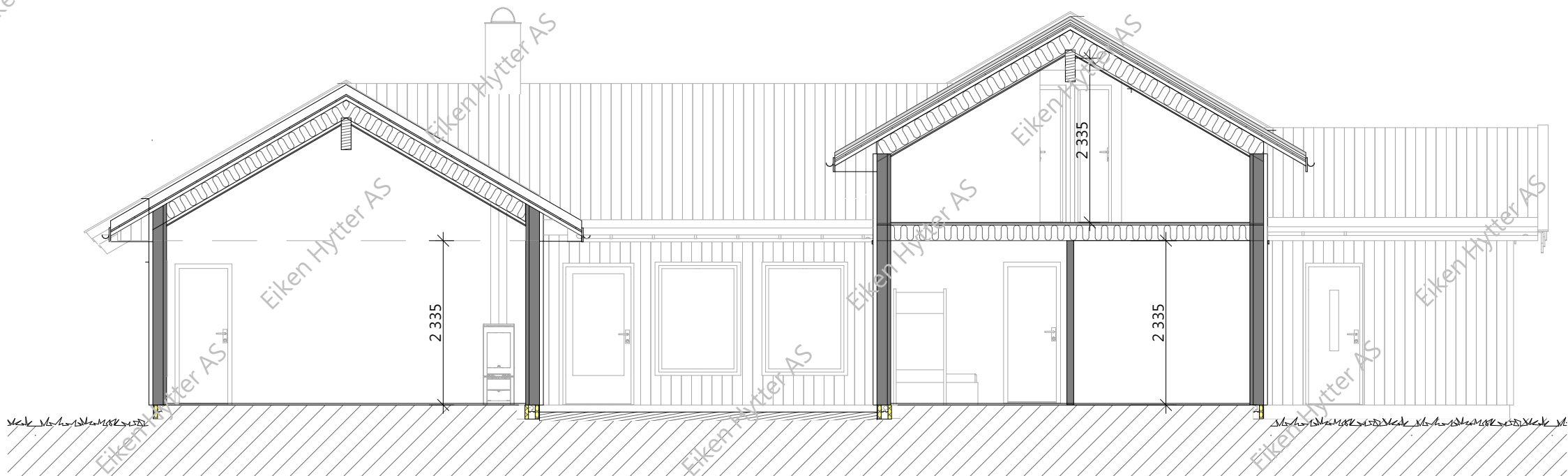
Snitt - B
