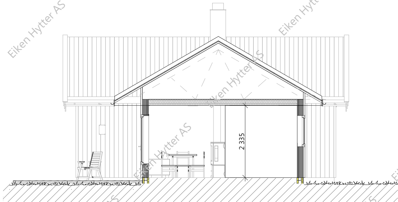
Snitt -A
