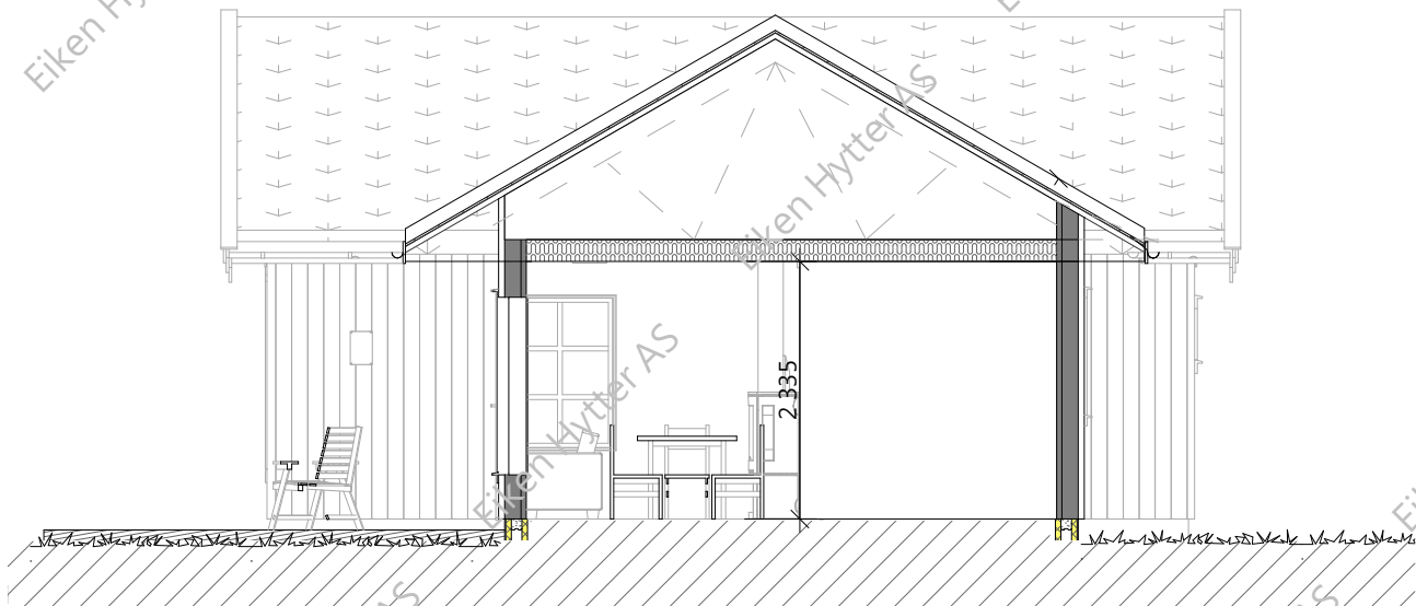
Snitt -A
