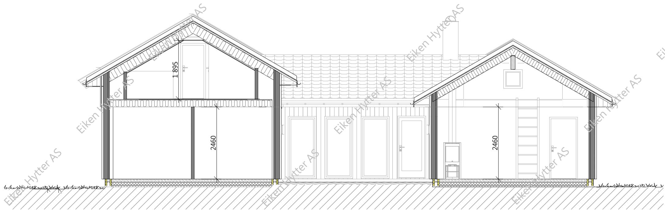
Snitt - A
