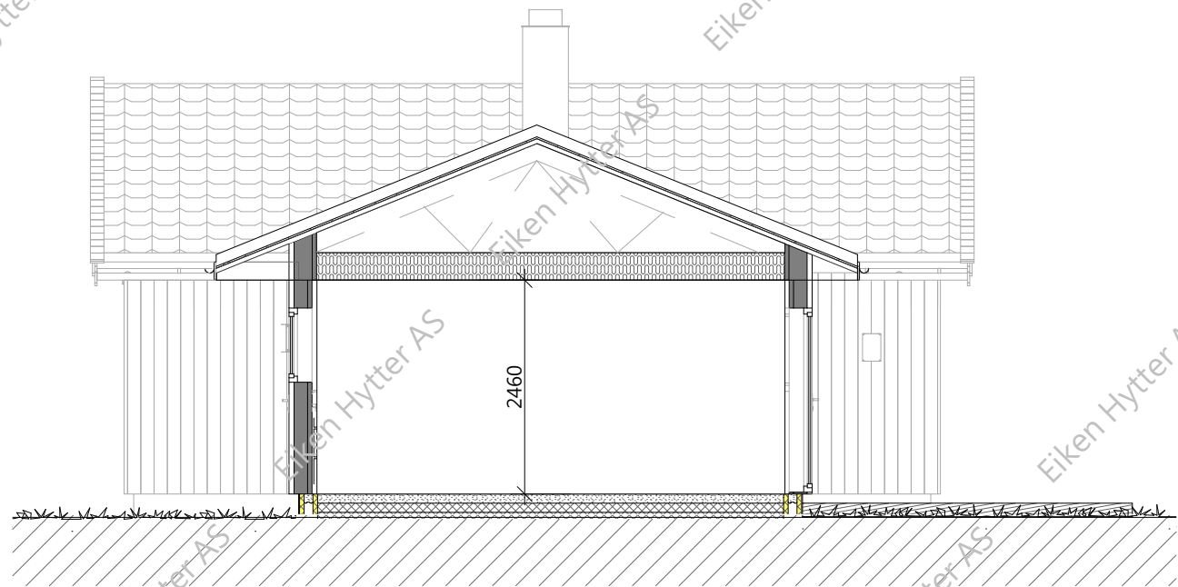
Snitt - A
