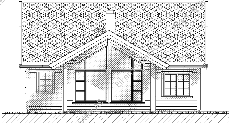
Fasade mot
