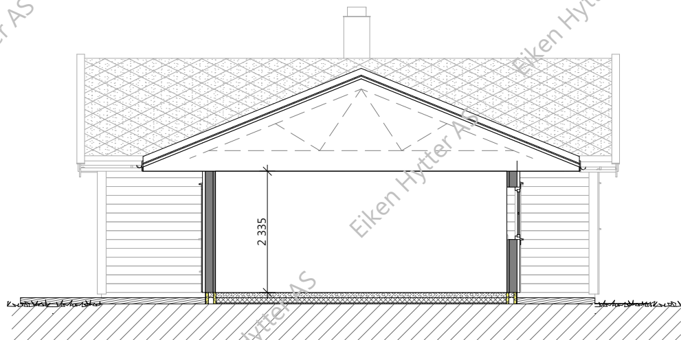
Snitt -A
