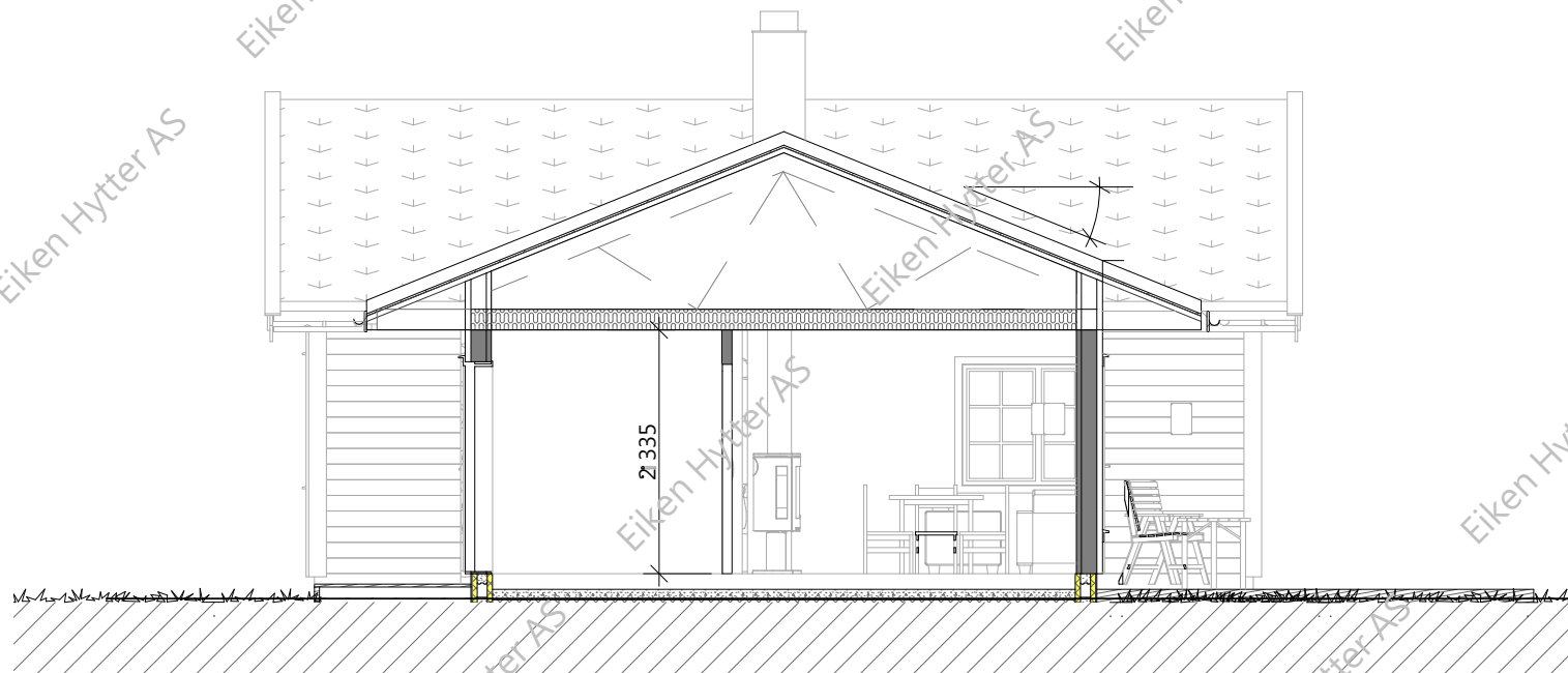
Snitt - B
