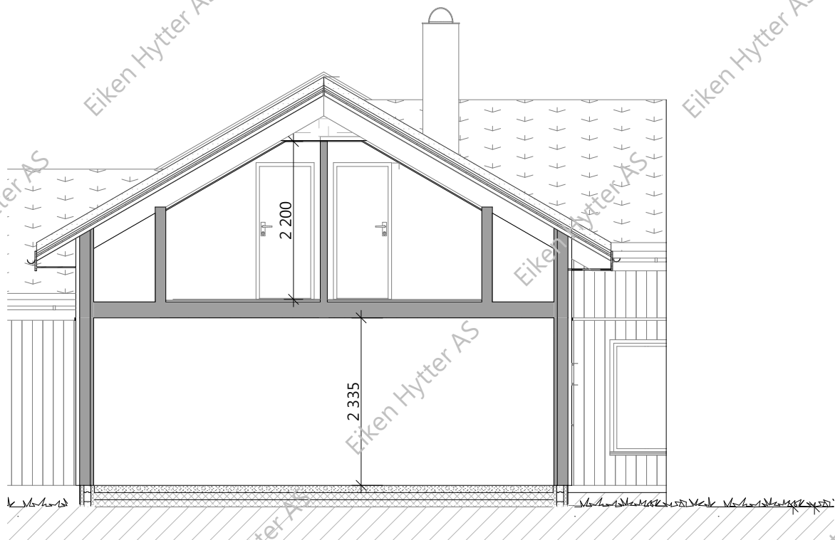
Snitt A - A
