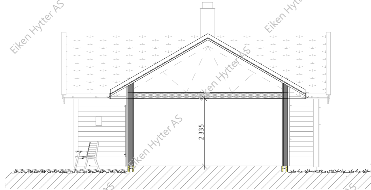
Snitt -A
