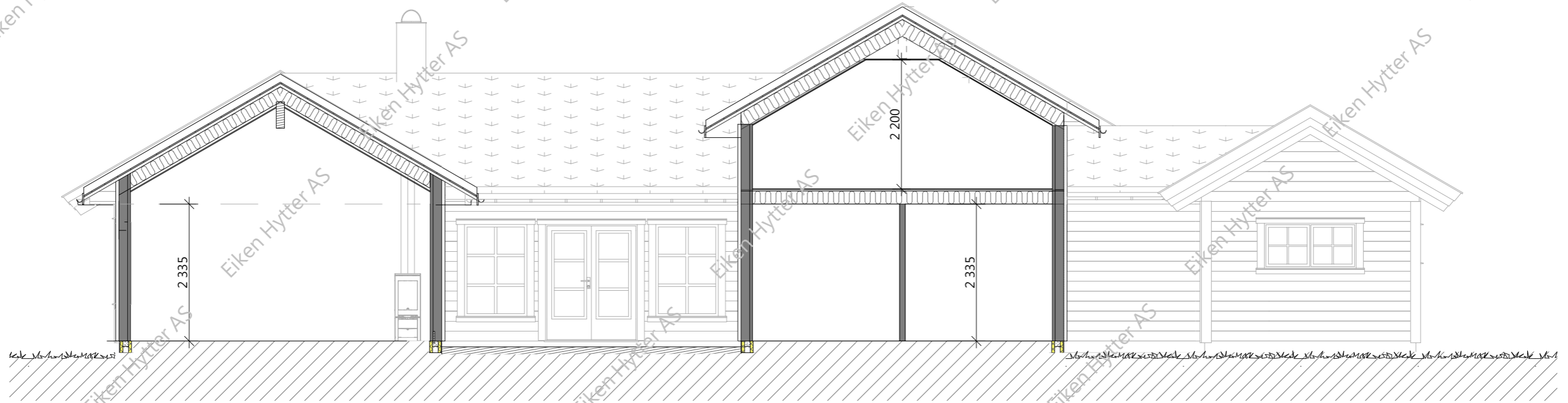
Snitt -A
