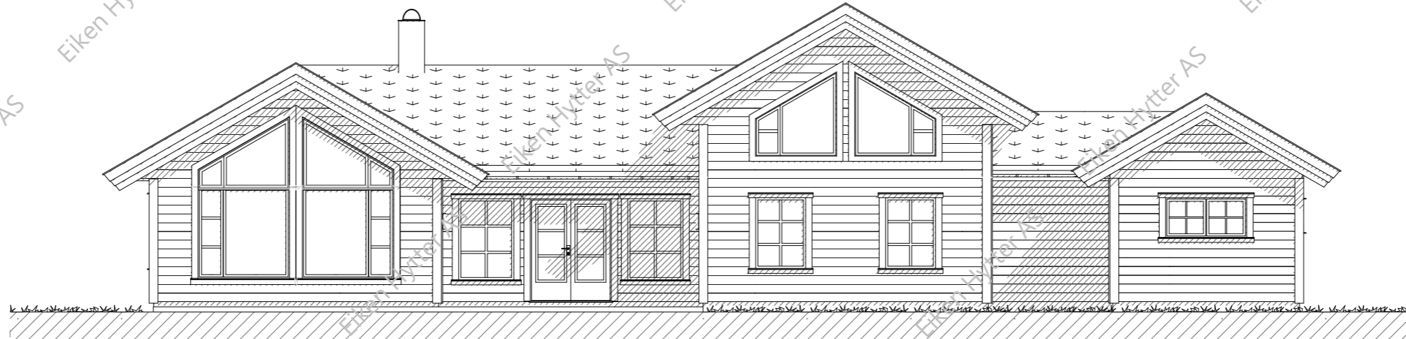
Fasade mot
