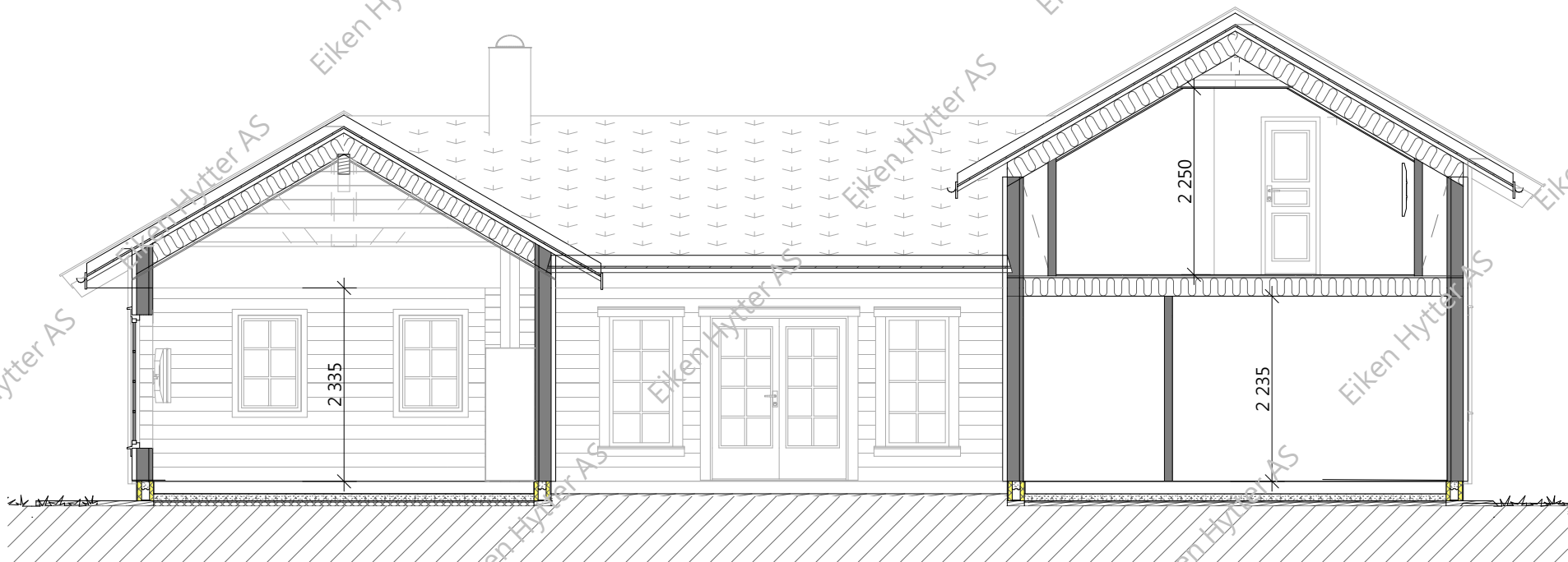
Snitt - B
