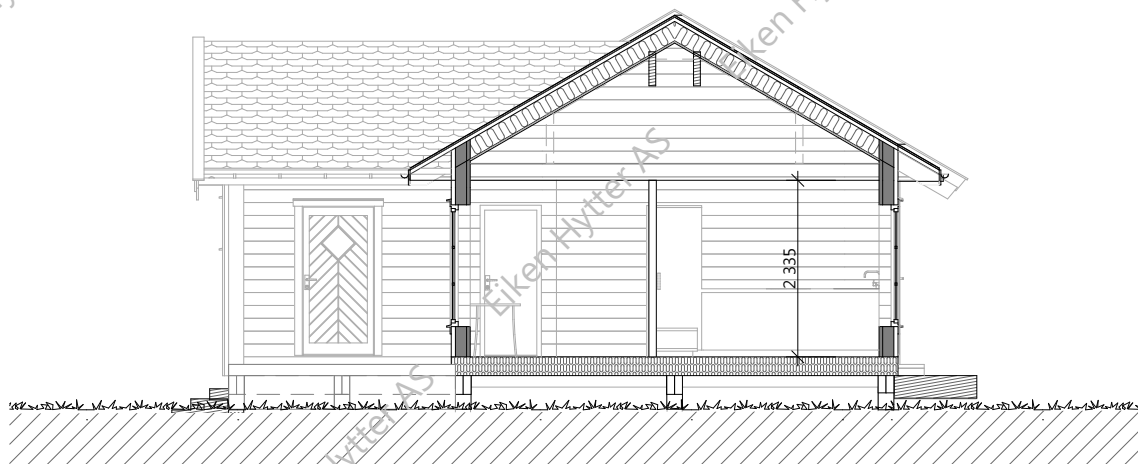
Snitt B-B
