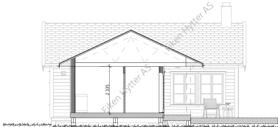
Snitt A-A
