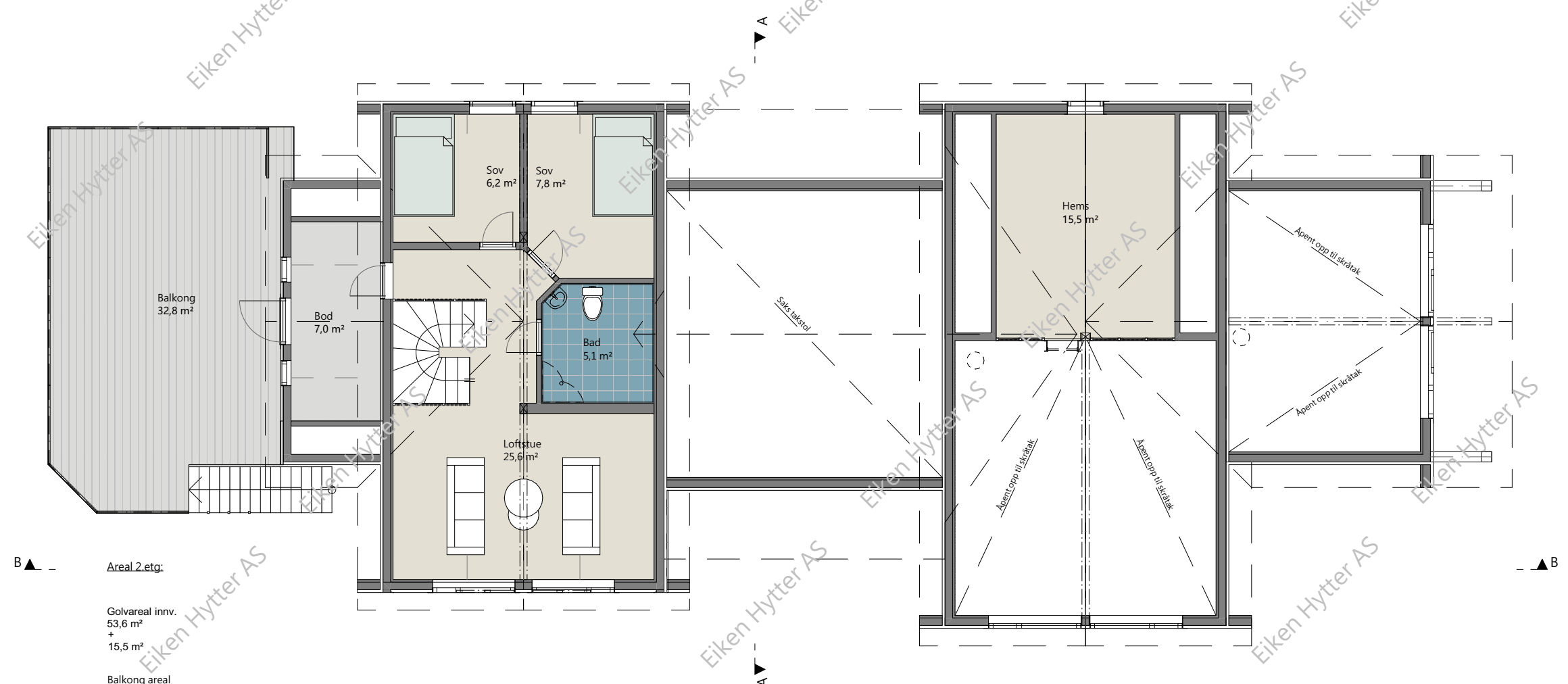
2. Etasje
