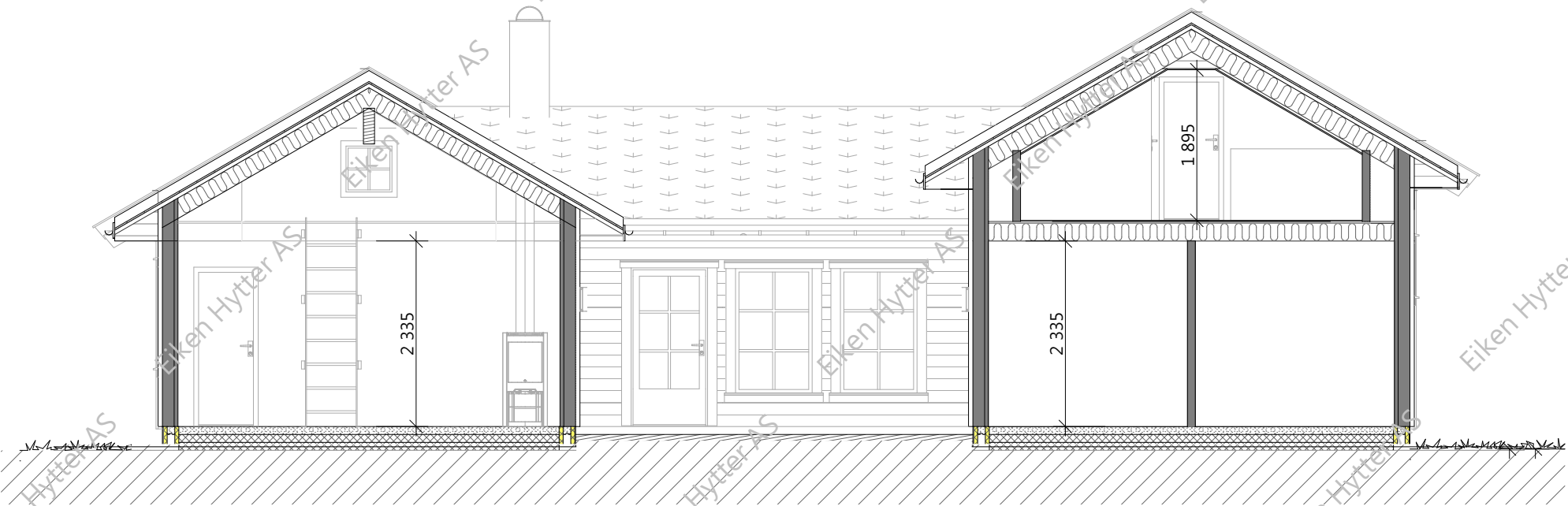
Snitt - A
