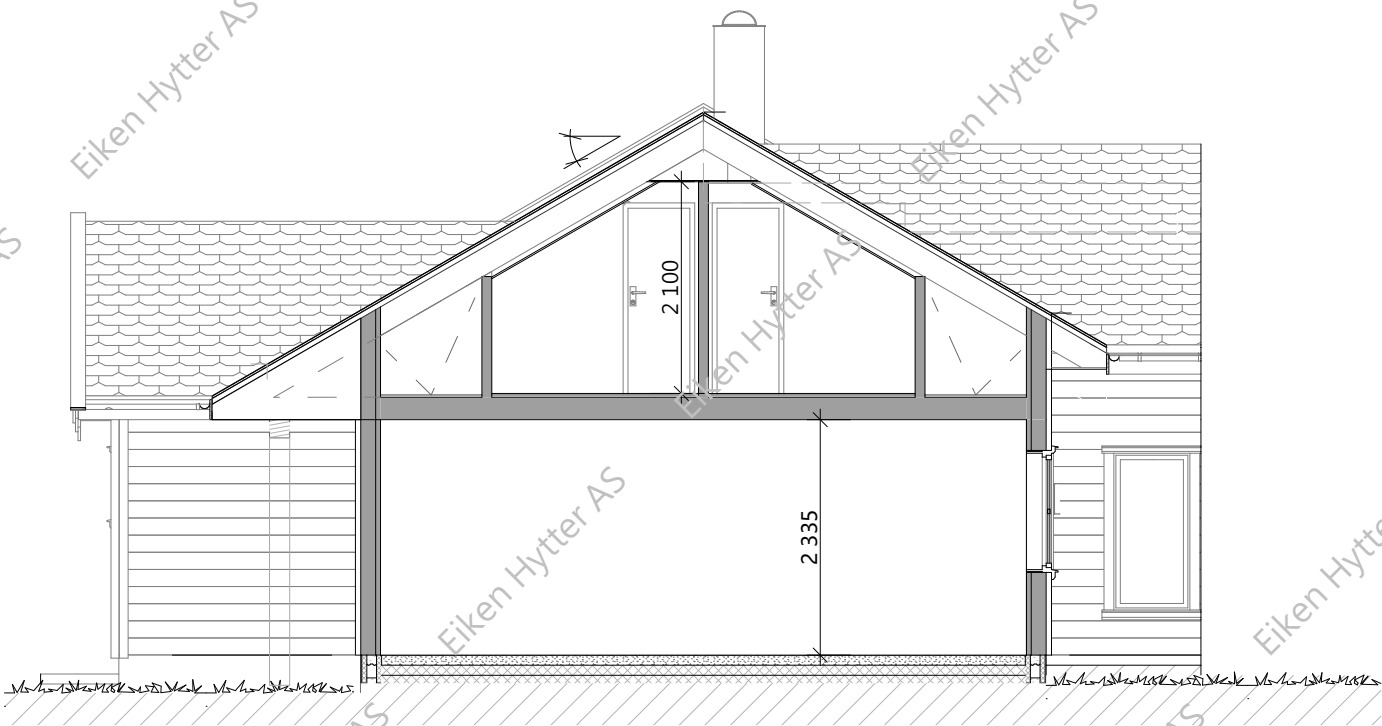
SNITT B
