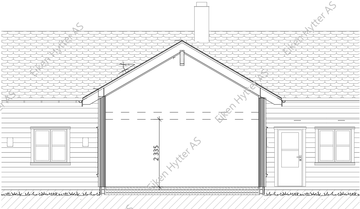
SNITT A
