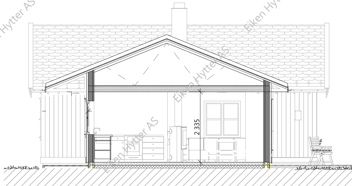
Snitt -A
