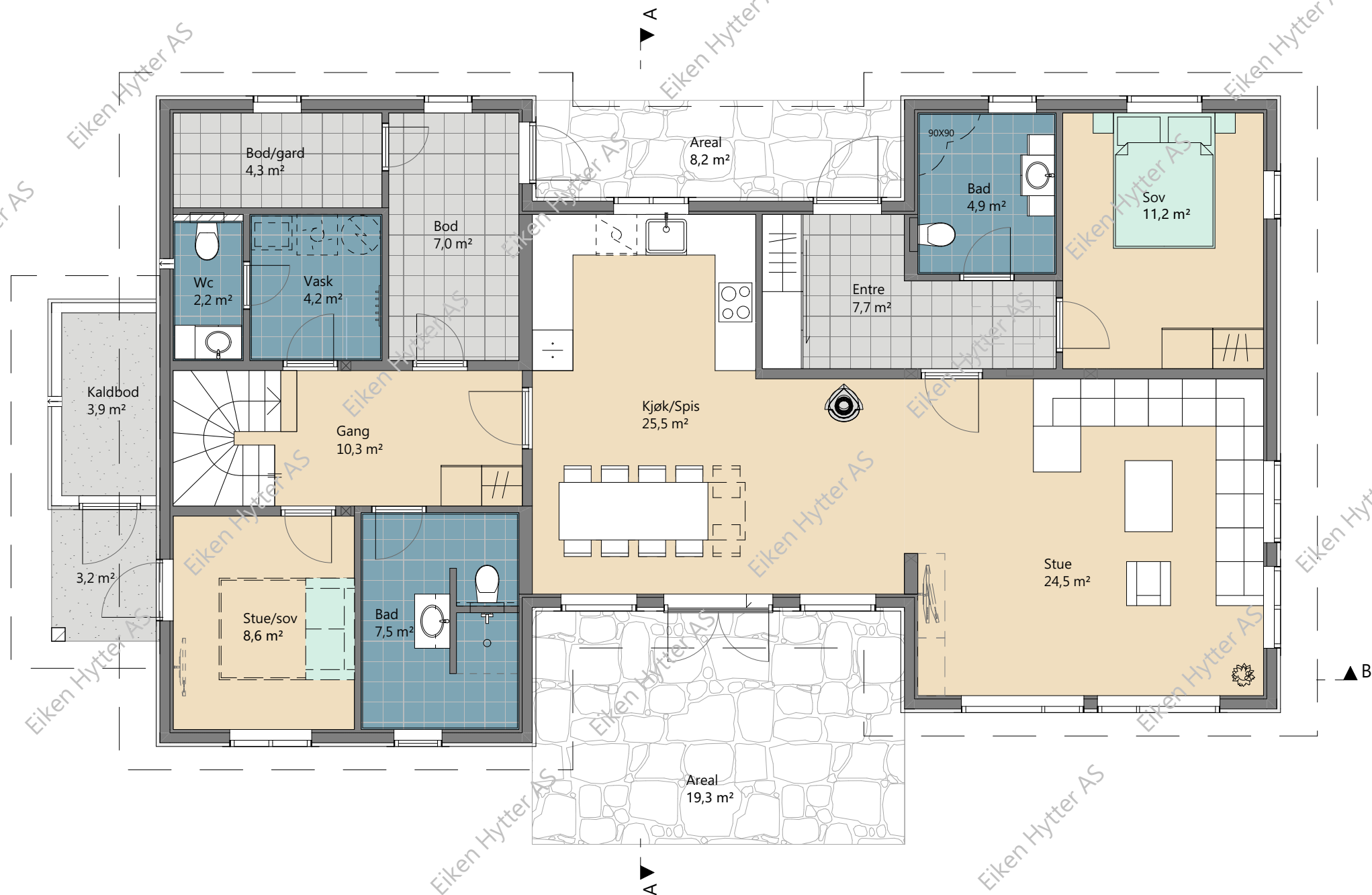
1. Etasje
