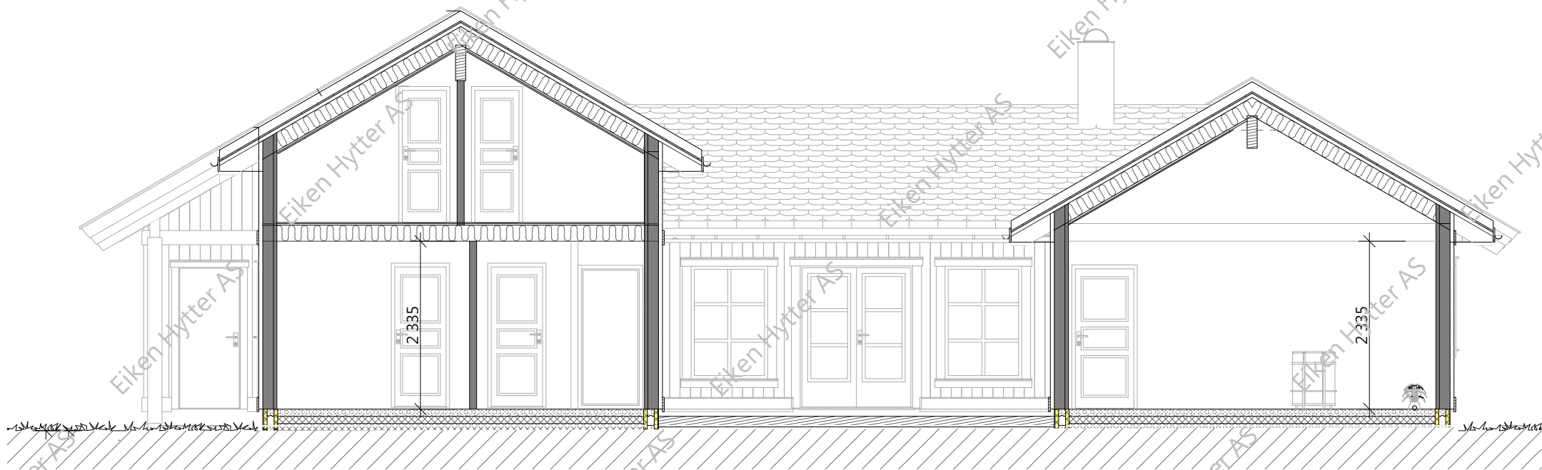
Snitt - B
