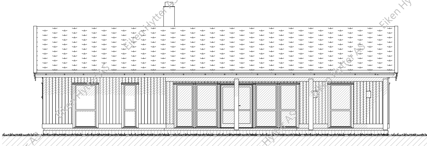
Fasade 1
