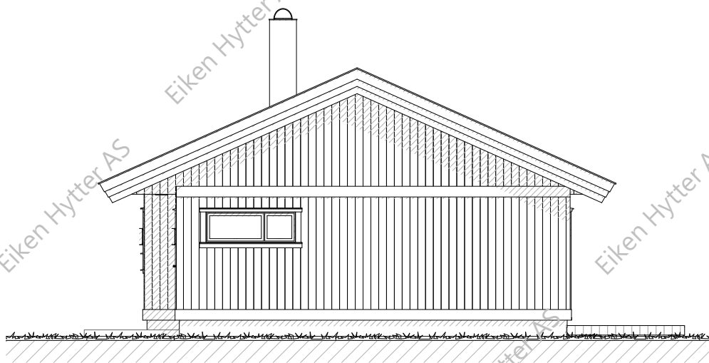
Fasade 3
