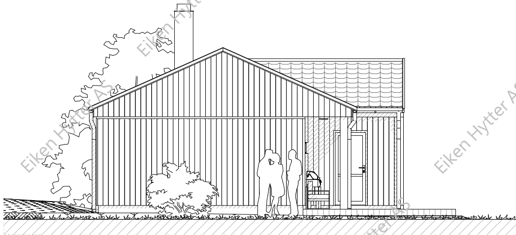
Fasade 3
