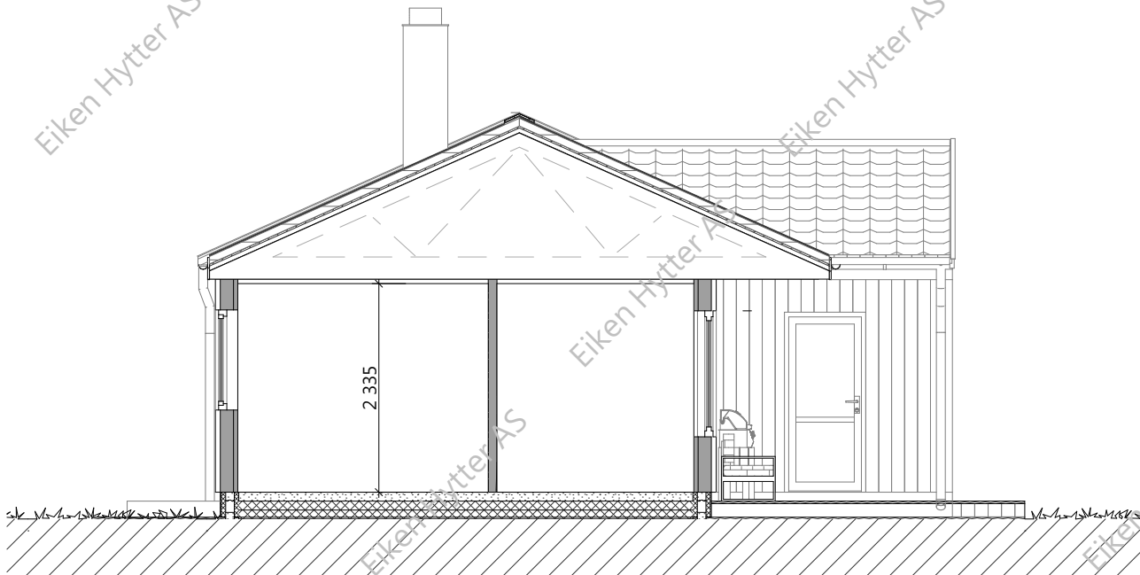
Snitt BB
