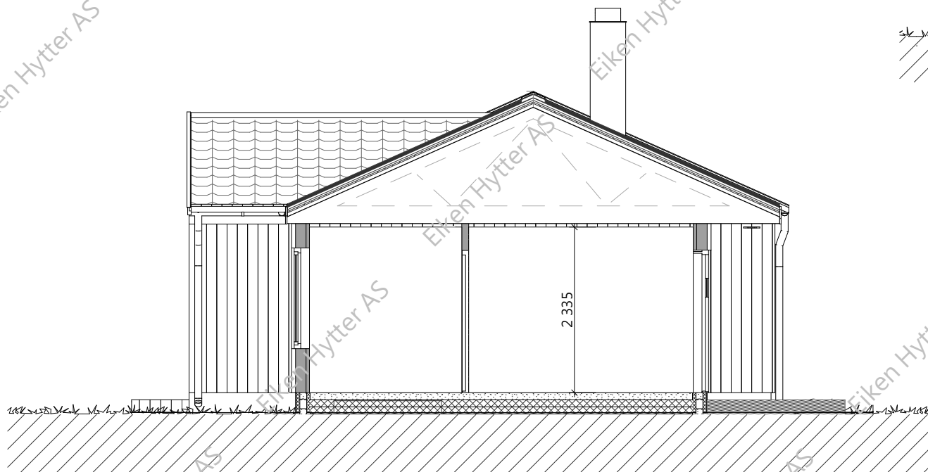
Snitt AA
