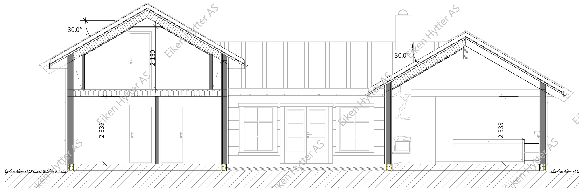
Snitt - A
