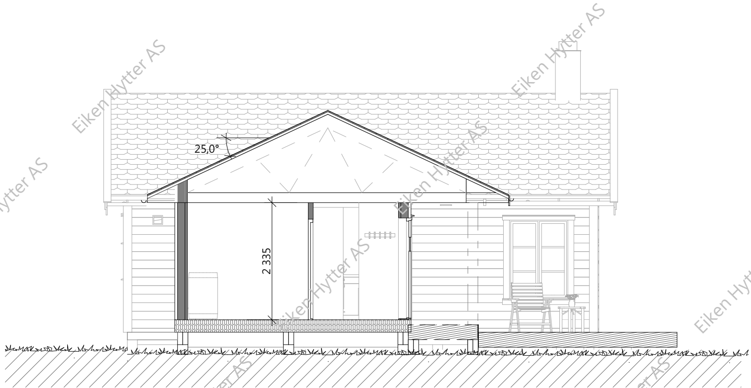
Snitt A-A
