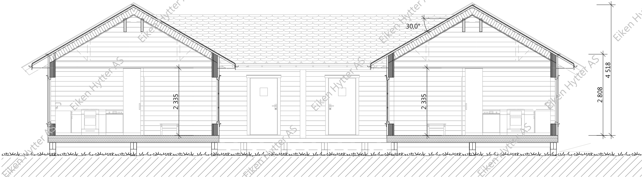
Snitt B-B
