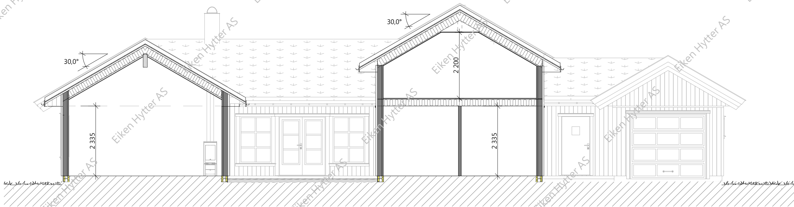
Snitt -A
