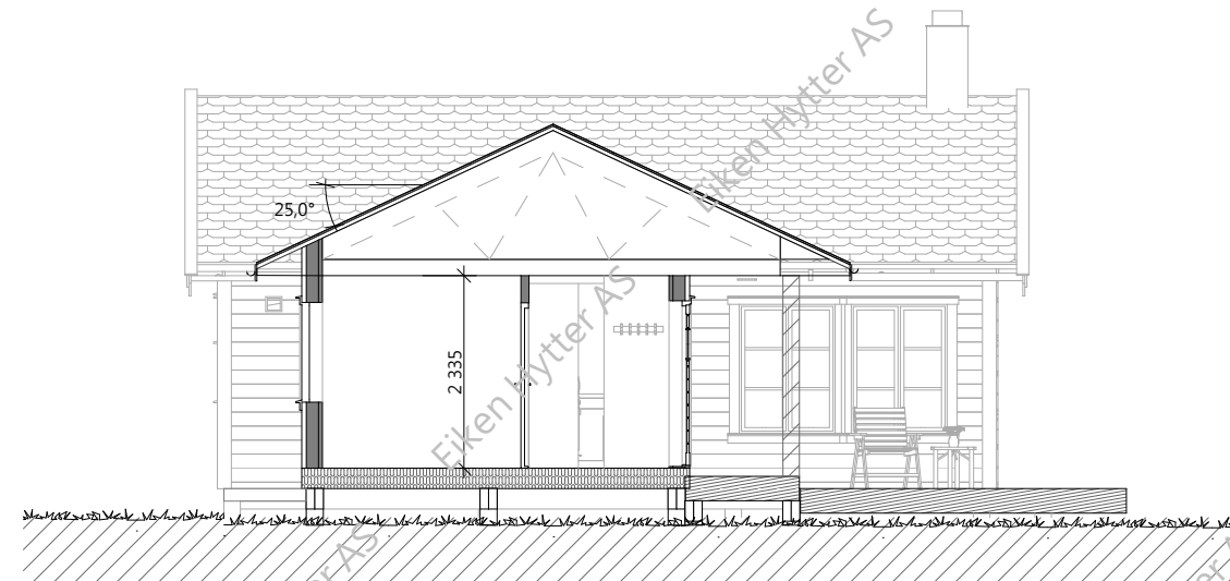
Snitt A-A
