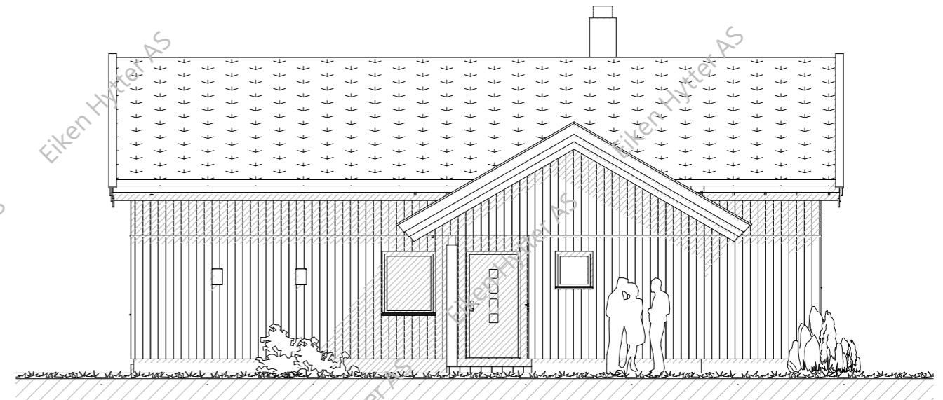
Fasade 4
