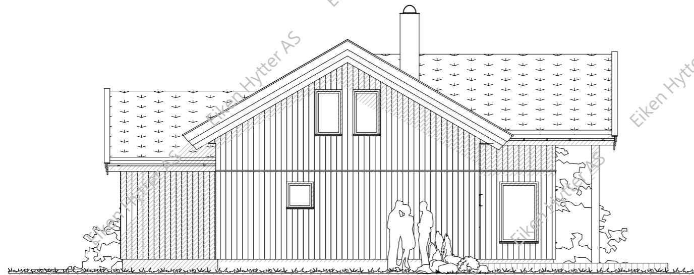
Fasade 3
