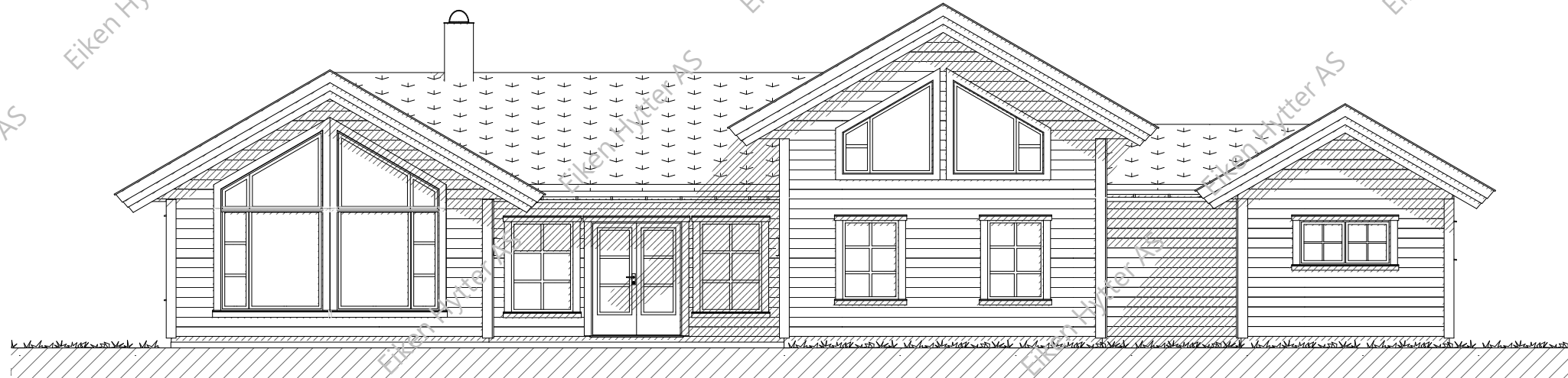
Fasade mot
