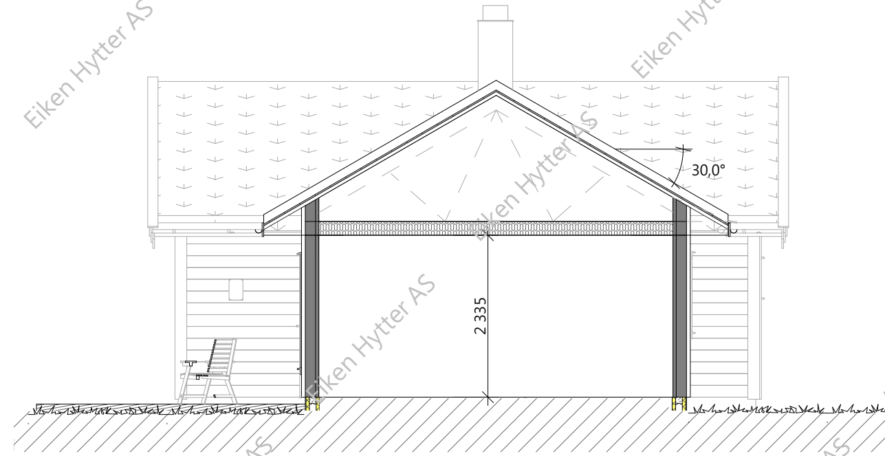
Snitt -A
