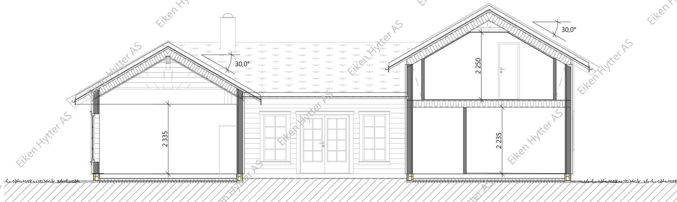
Snitt - B
