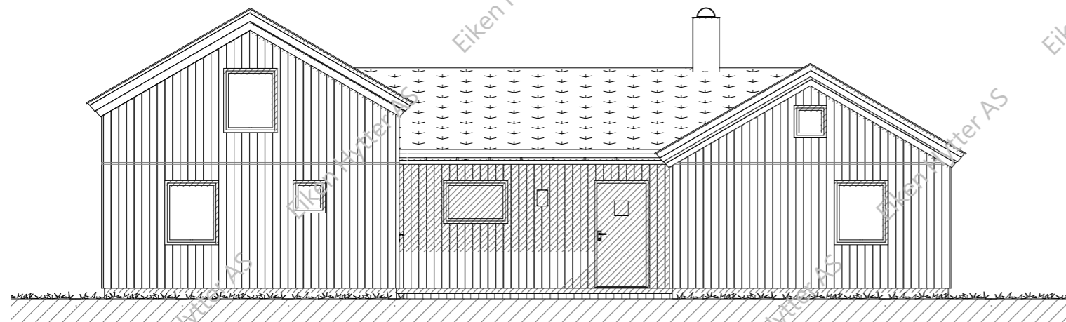
Fasade 3
