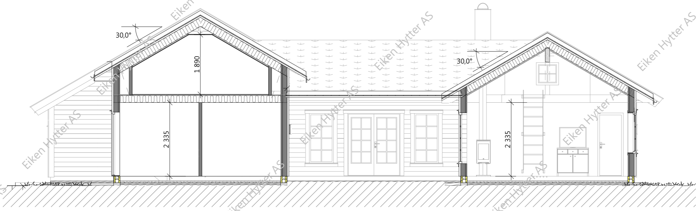
Snitt - B
