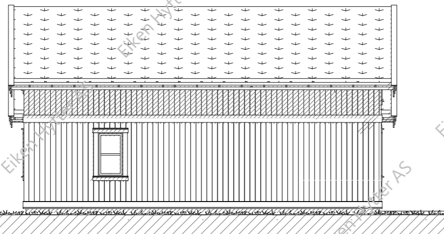
Fasade 2
