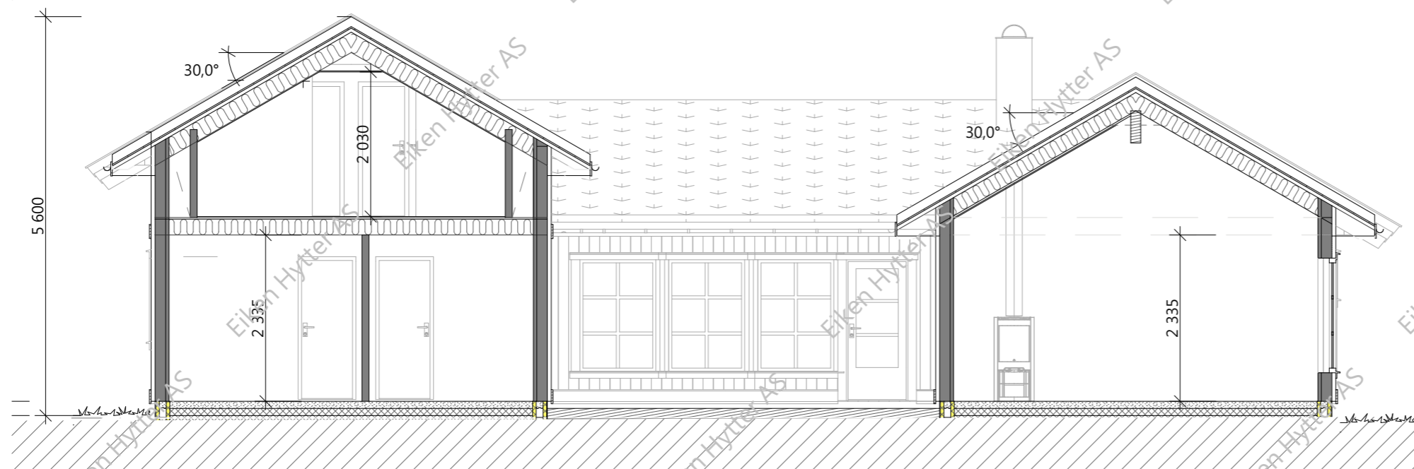
Snitt - A
