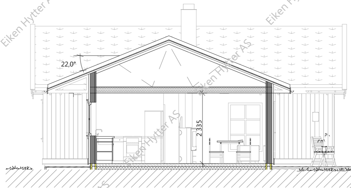
Snitt - A
