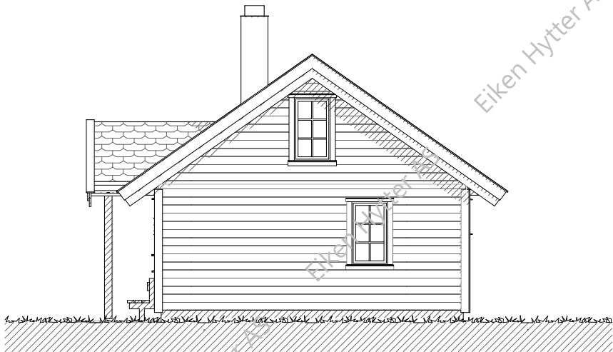
Fasade 4
