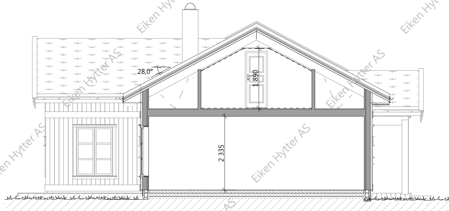
Snitt A - A
