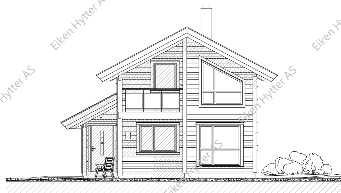
Fasade 2
